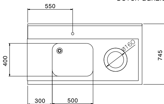
Boven aanzicht
